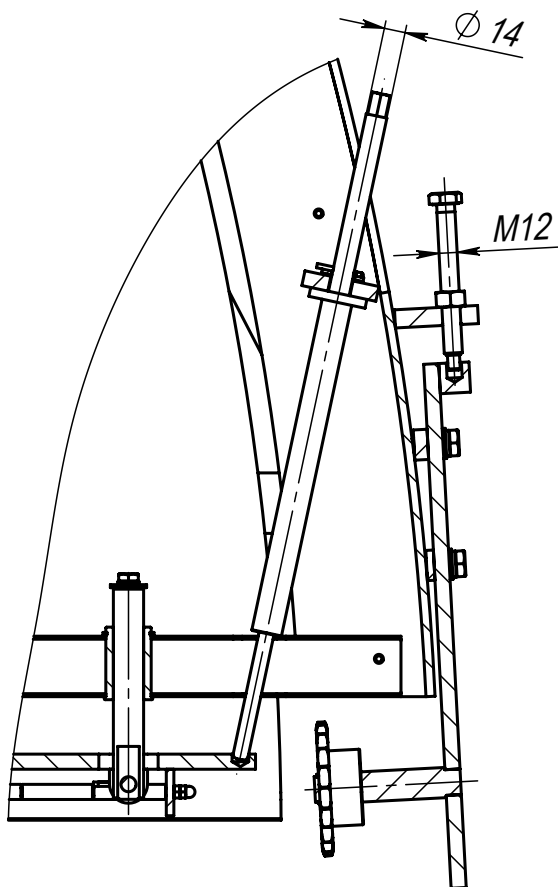
В-В (1 : 5) Натяжение ленты
