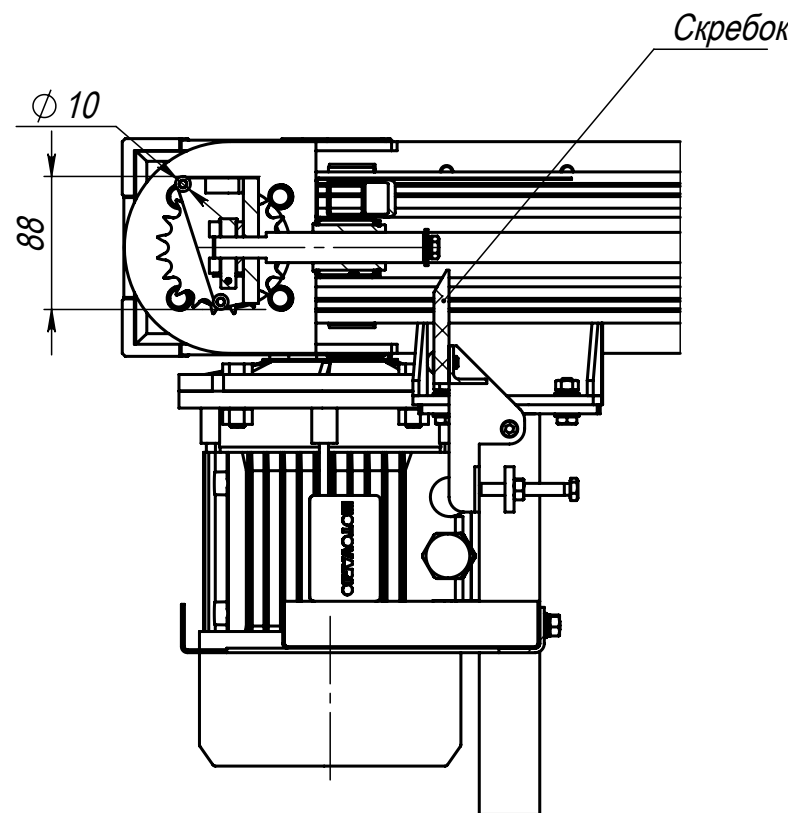
Б-Б (1 : 5)
