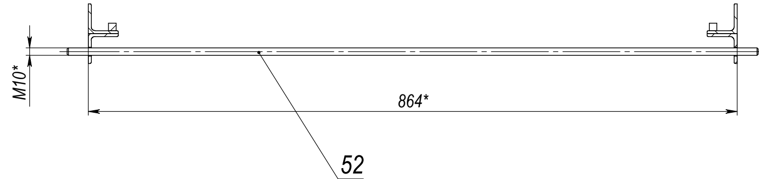
Е(1:5)(1)
