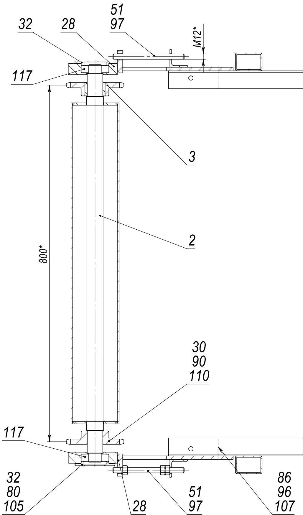
Б-Б(1:5)(1)
