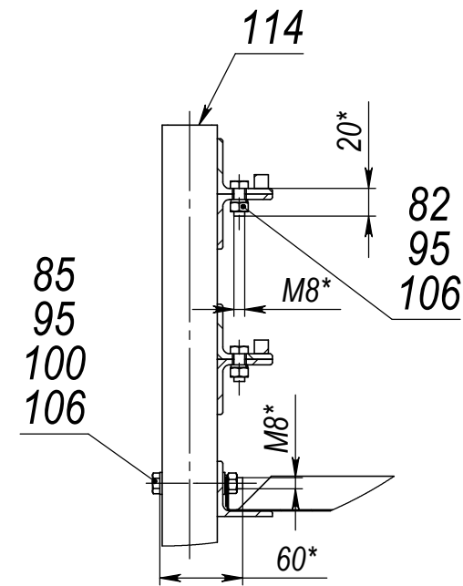
Ж-Ж(1:5)(1)
