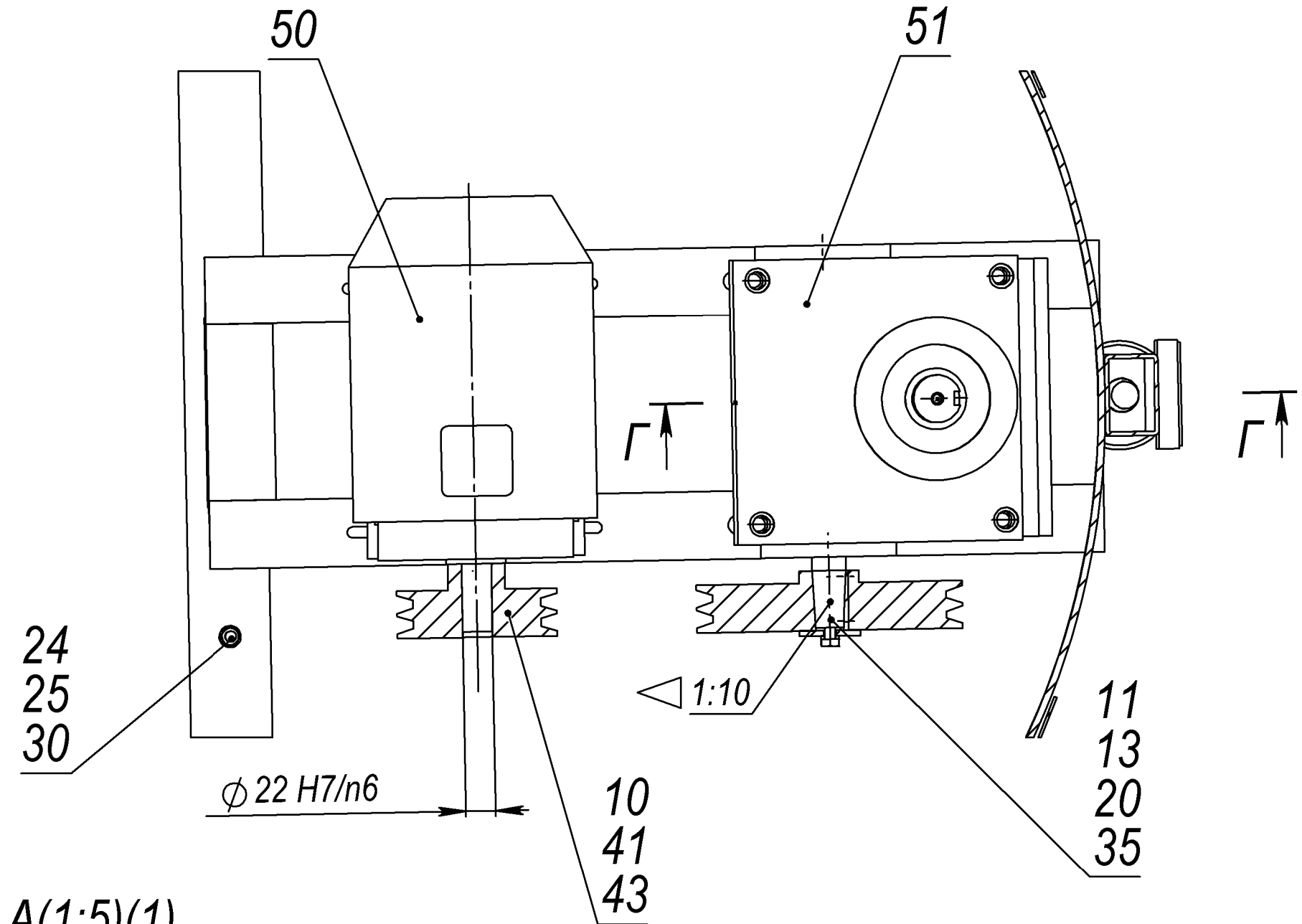
Б-Б(1:4)
