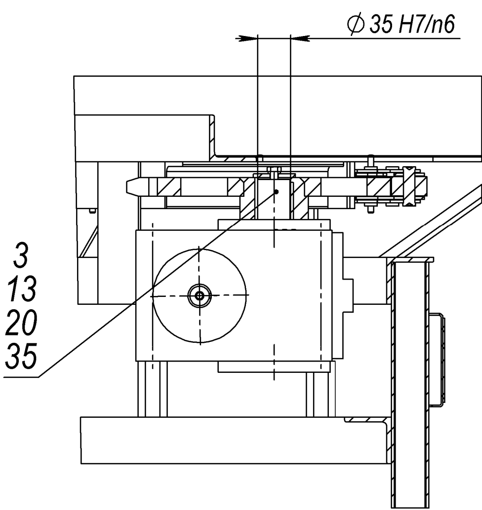
Г-Г (1 : 4)
