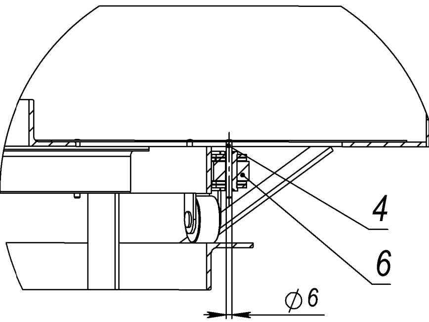
Д-Д(1:4)(1)
