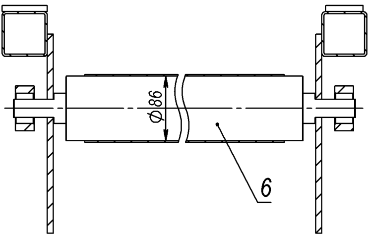
Д-Д (1 : 5)
