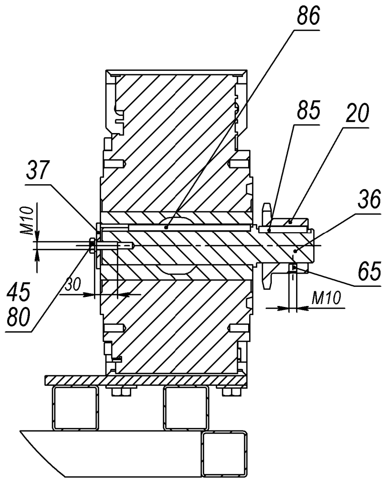
И-И (1 : 5)
