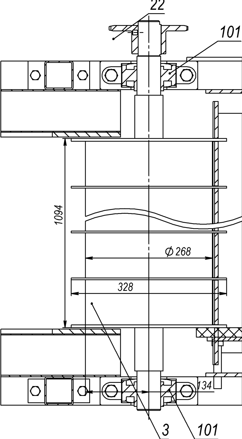
В-В (1 : 5)
