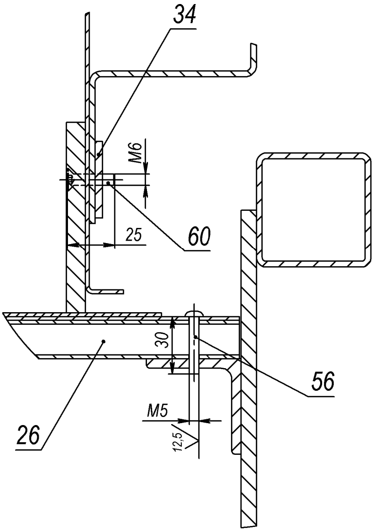
Л-Л (1 : 2)
